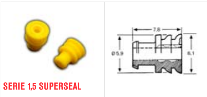
TAPÓN DE CIERRE SERIE 1,5 SUPERSEAL
